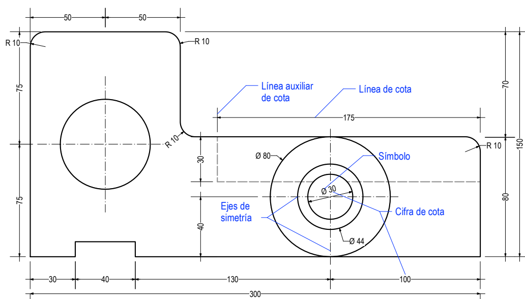
Fig. 11 Ejemplo de acotación de una pieza, en mm
