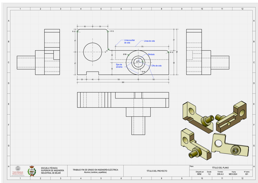
Fig. 3 Cajetín recomendado para un formato apaisado (DIN A3)
